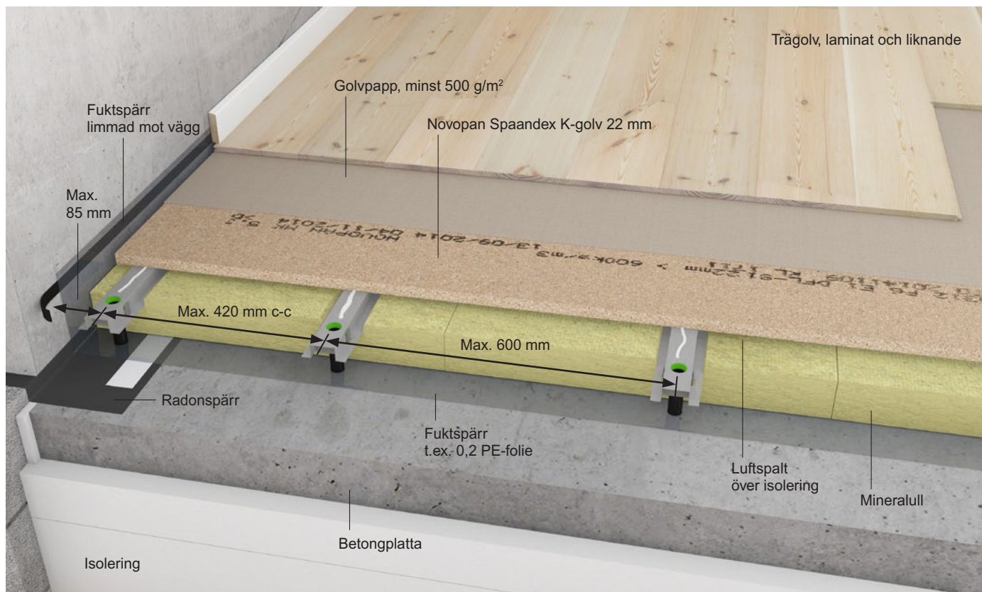
Figur 1 Novopan Spaandex K-golv 22 mm på stålreglar – system Granab 3000N. Reglarna monteras med kantreglar längs alla väggar och et regelavstånd i första facket längs väggarna på 420 mm c-c.
